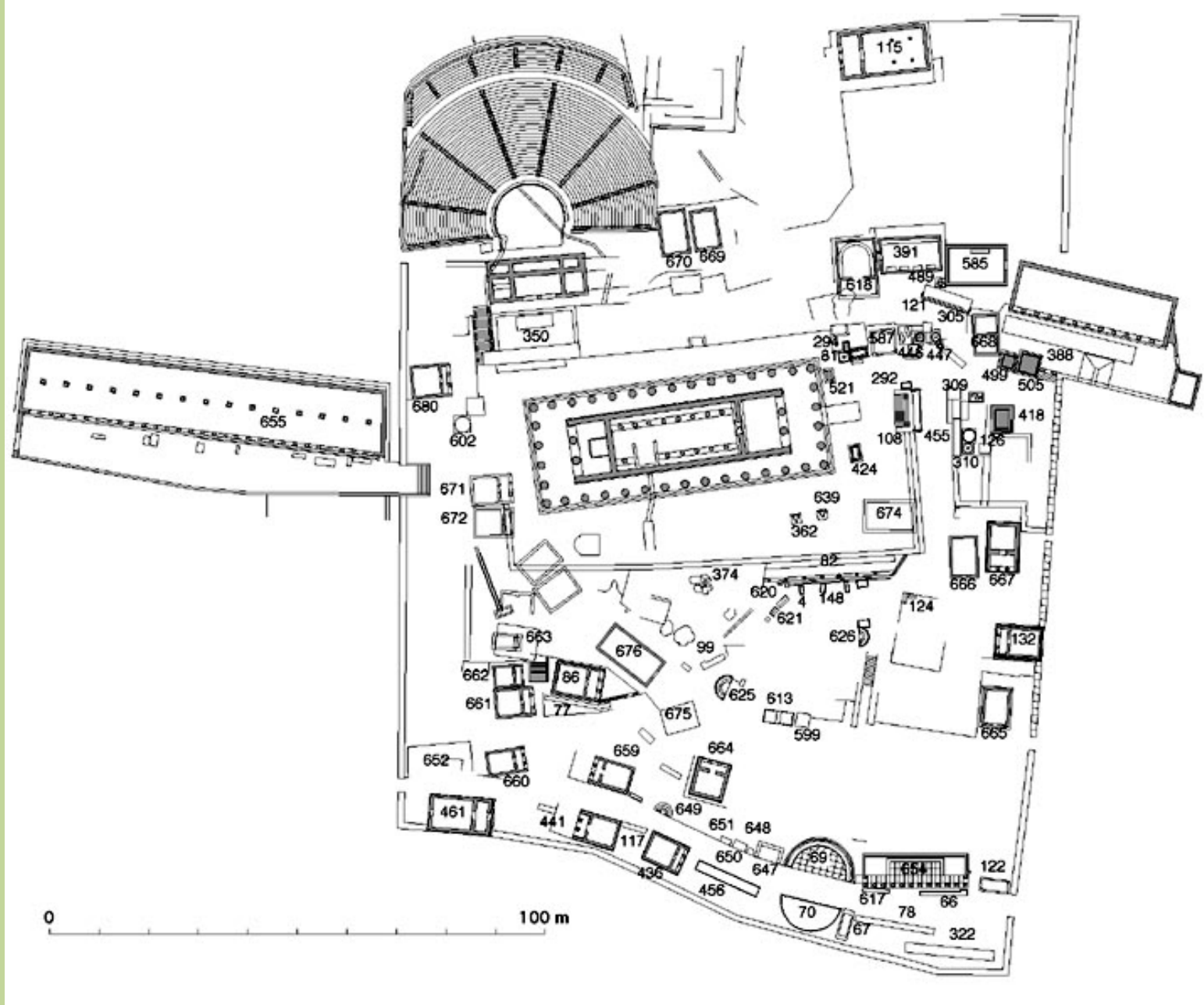
Plan général du sanctuaire de Delphes.
