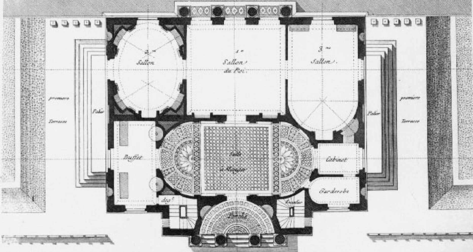
Plan du Rez-de-Chaussée du Pavillon de Louveçiennes.
